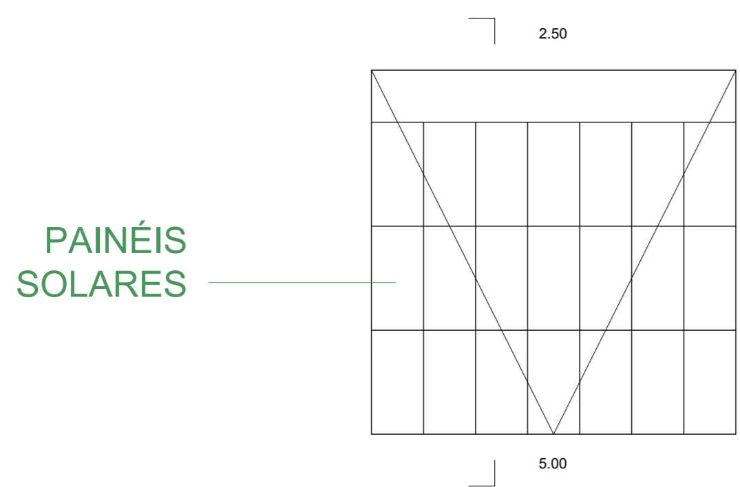
PLANTA COBERTURA
